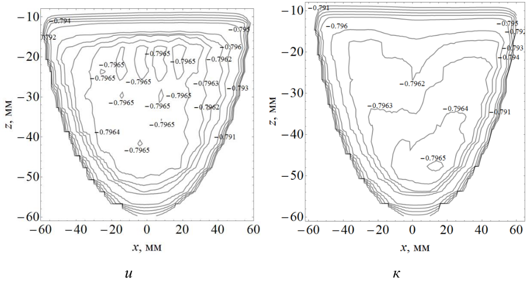
Рис. 12. Распределение магнитного поля в медианной плоскости вдоль осей z и x полюса 1 (а, б), полюса 2 (в, г), полюса 3 (д, е), полюса 4 (ж, з). Один из двух магнитов назван D1, другой – D2. Карты магнитного поля в медианной плоскости в области основного полюса магнита D1 (и) и D2 (к)
