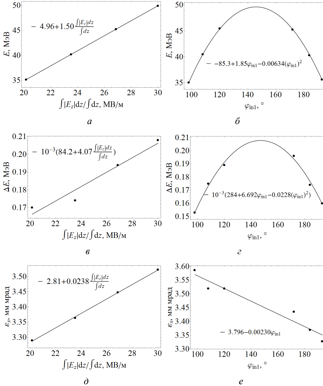
Рис. 5. Средняя кинетическая энергия E (а, б), полный разброс кинетических энергий частиц пучка \Delta E (в, г), нормализованный поперечный эмиттанс \epsilon_x (д, е) пучка после ускорения в линейном ускорителе при регулировании конечной энергии методом 1 с помощью нормировки поля \int |E_z| dz / \int dz (слева) и методом 2 с помощью фазы влета в первую секцию \varphi_{in1} (справа)
