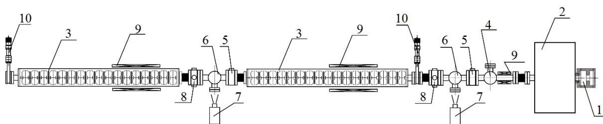
Рис. 1. 1 – СВЧ пушка, 2 – соленоид, 3 – секции линейного ускорителя, 4 - камера ввода лазерного импульса, 5 – датчик заряда, 6 – камера флуоресцентного экрана, 7 – ПЗС камера, 8 – датчик положения пучка, 9 – корректоры пучка, 10 – вакуумный затвор
