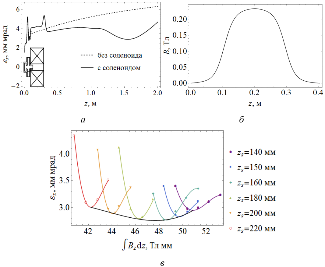
Рис. 3. (а) Изменения нормализованного поперечного эмиттанса \epsilon_x при наличии магнитного поля соленоида: z_s = 200 мм, \int B_z dz = 44.3 Тл мм. (б) Распределение магнитного поля на оси соленоида. (в) Наименьший нормализованный поперечный эмиттанс пучка \epsilon_x при разных положениях соленоида z_s и интегралах его магнитного поля \int B_z dz
